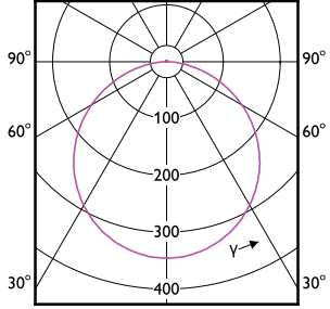
(cd/1000lm) 0°
